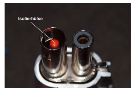
Foto. 7.4.24 EBERL plug
