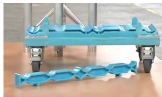
Foto 10.0-1 Truss dolly
