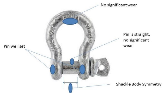
Foto 10.2-19 checking shackles
