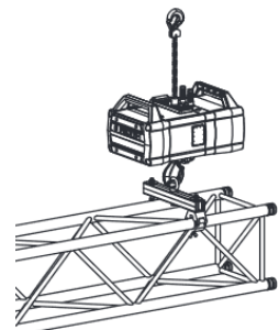
Foto 10.3-13 Chain hoist
