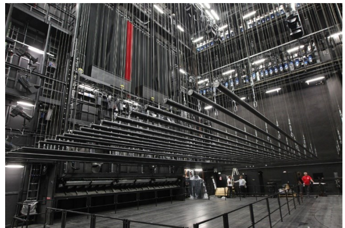
Foto 10.3-7 Fly bars
