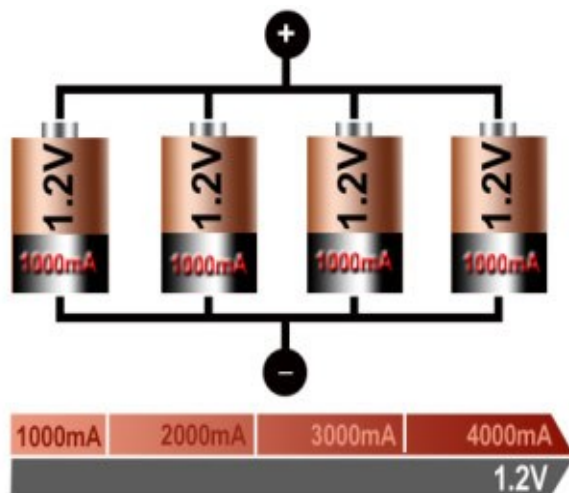
Dia 7.1.7 Parallelschakeling van batterijen
