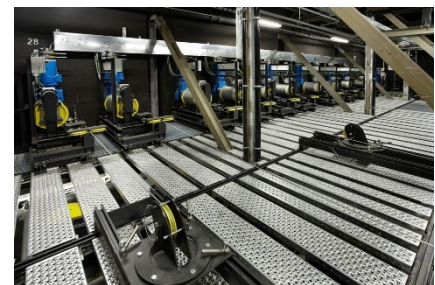
Foto 10.3-12 Point hoists
